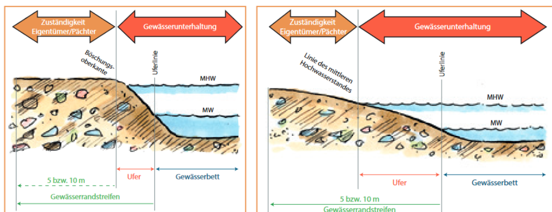
Abb. Zuständigkeit und Unterhaltungspflicht an Gewässern mit ausgeprägter Böschungsoberkante (links) und ohne ausgeprägte Böschungsoberkante (rechts) (MW= Mittelwasserstand, MHW= mittleres Hochwasser) (Grafik: Büro am Fluss)
