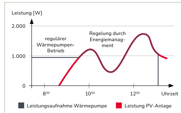
Grafik 2: Die Leistung der Wärmepumpe passt sich dynamisch an die erzeugte PV-Strommenge an.
