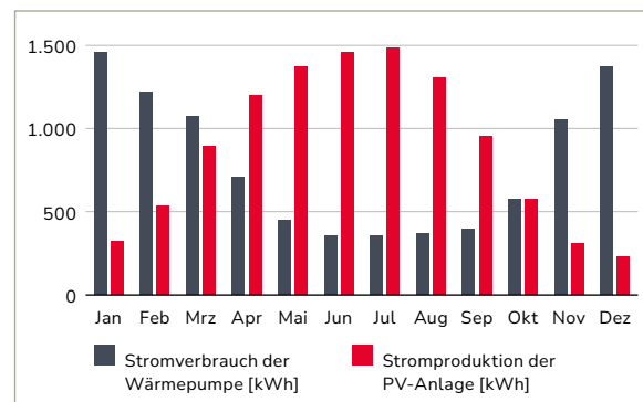
Grafik 1: Monatlicher Wärmepumpen-Stromverbrauch und monatliche PV-Stromproduktion im Jahresverlauf
