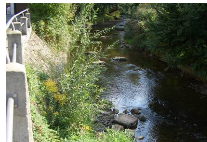
struktureicher Böschungsfuß auf engem Raum (Losse, Kassel)
