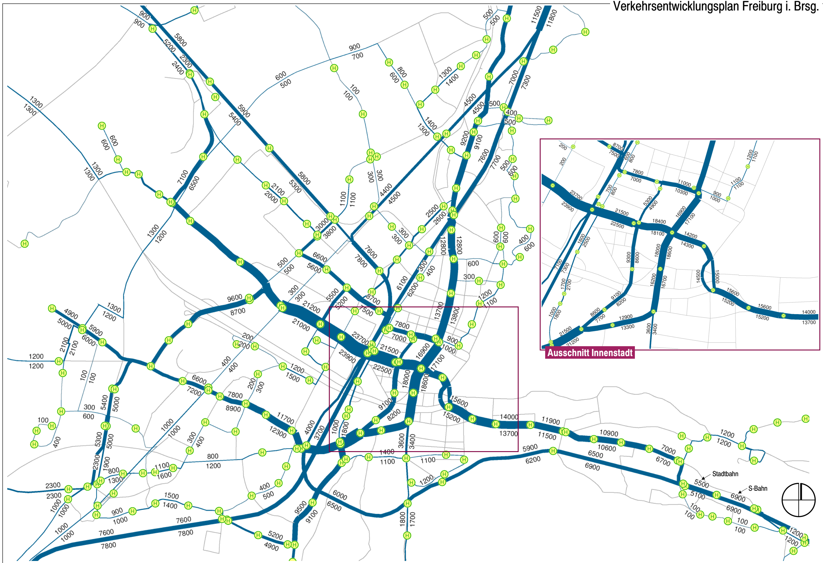
Verkehrsaufkommen ÖPNV Planfall "Maßnahmenprogramm 2020" Personenfahrten / 24h (Grundlage: Modellrechnung)
