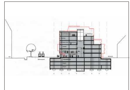
Schnitt, Entwurf Universitätsbauamt Freiburg
